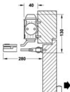
Montage standard corps sur porte, pose côté paumelles
